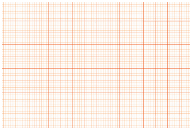
Слика 2. Масени удео соли у засићеном раствору на различитим температурама
