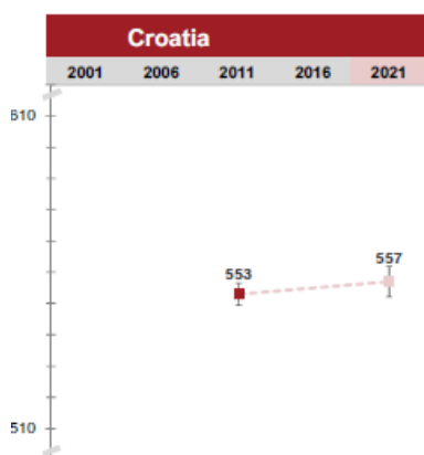
Slika 1. Trend u prosječnim rezultatima 2011. – 2021.
